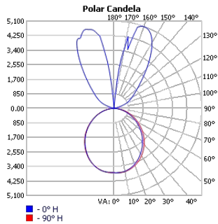
TECHOLED-ASY-DI-63-HI-30
