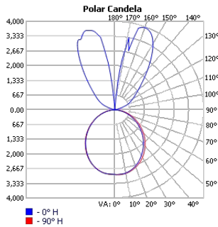
TECHOLED-ASY-DI-63-ME-30
