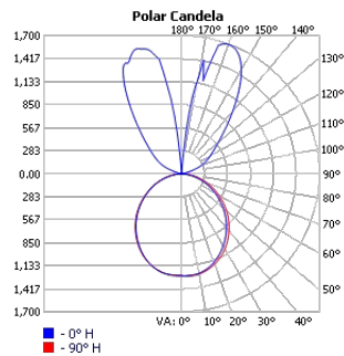
TECHOLED-ASY-DI-42-LO-30
