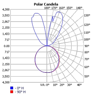
TECHOLED-ASY-DI-42-HI-30
