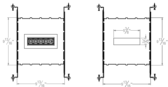
Dimensions
