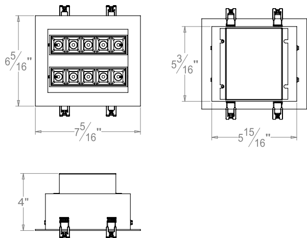
Dimensions
